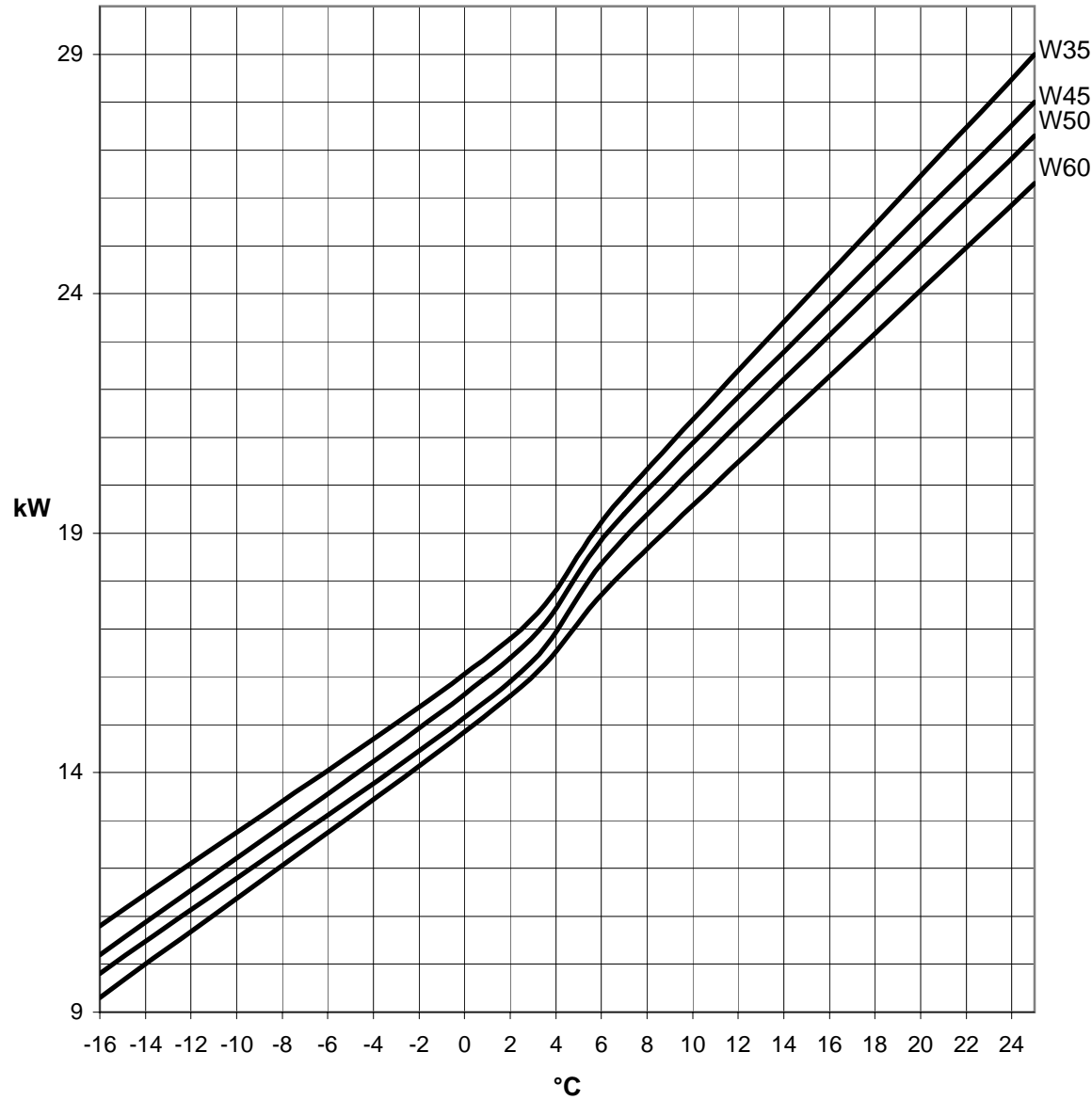
Heizleistung GMLW 19 plus
