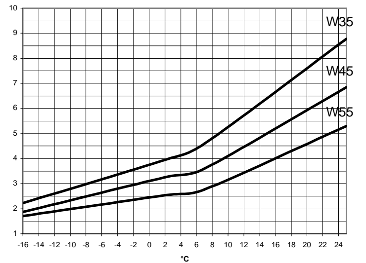
Leistungszahl GMLW 19
