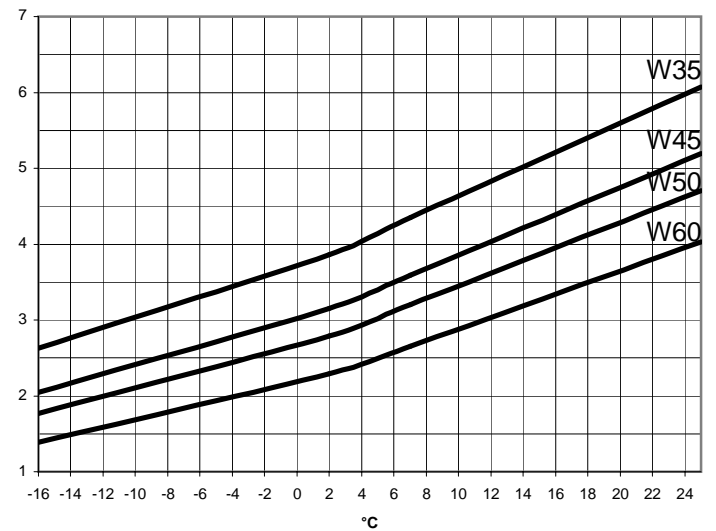
Leistungszahl GMLW 9 plus
