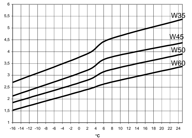
Leistungszahl GMLW 19 plus
