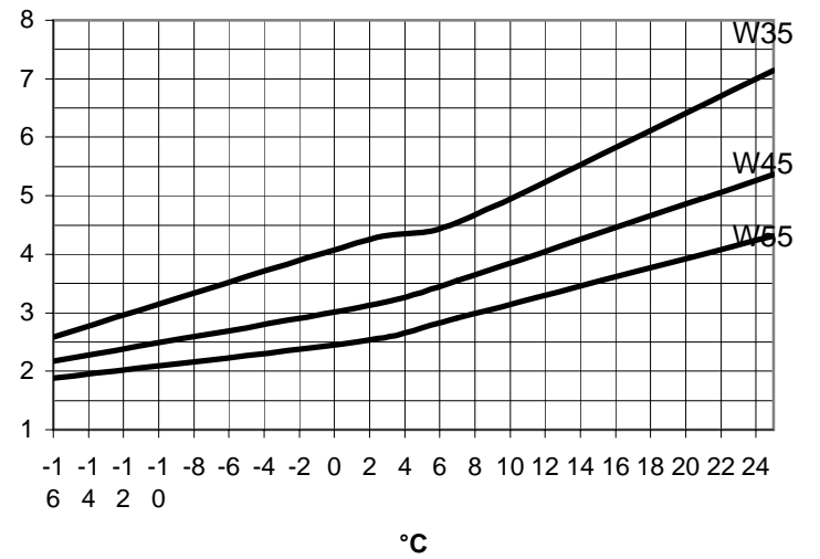
Leistungszahl GMLW 9
