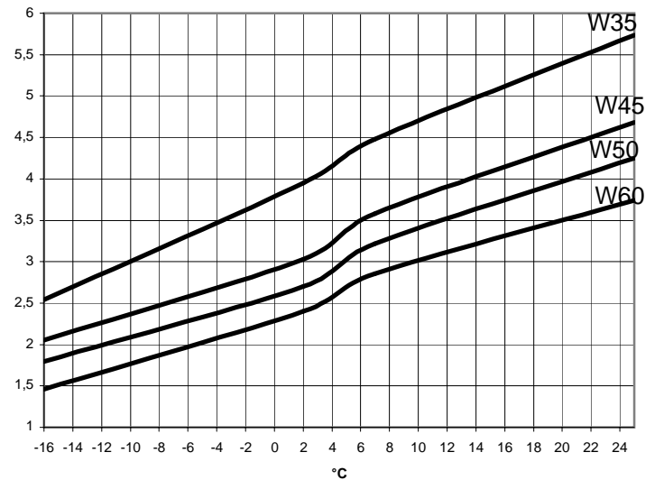
Leistungszahl GMLW 25 plus
