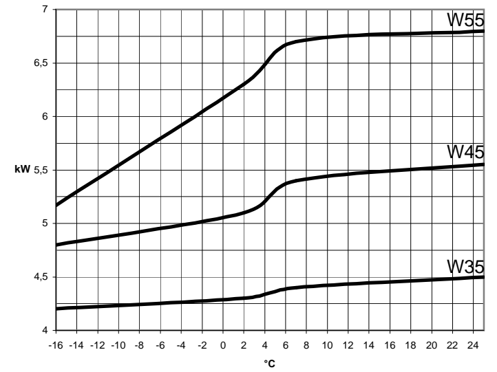
Leistungsaufnahme GMLW 19
