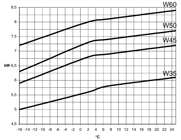
Leistungsaufnahme GMLW 25 plus
