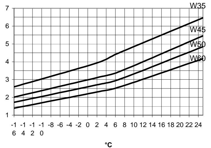
Leistungszahl GMLW 35 plus
