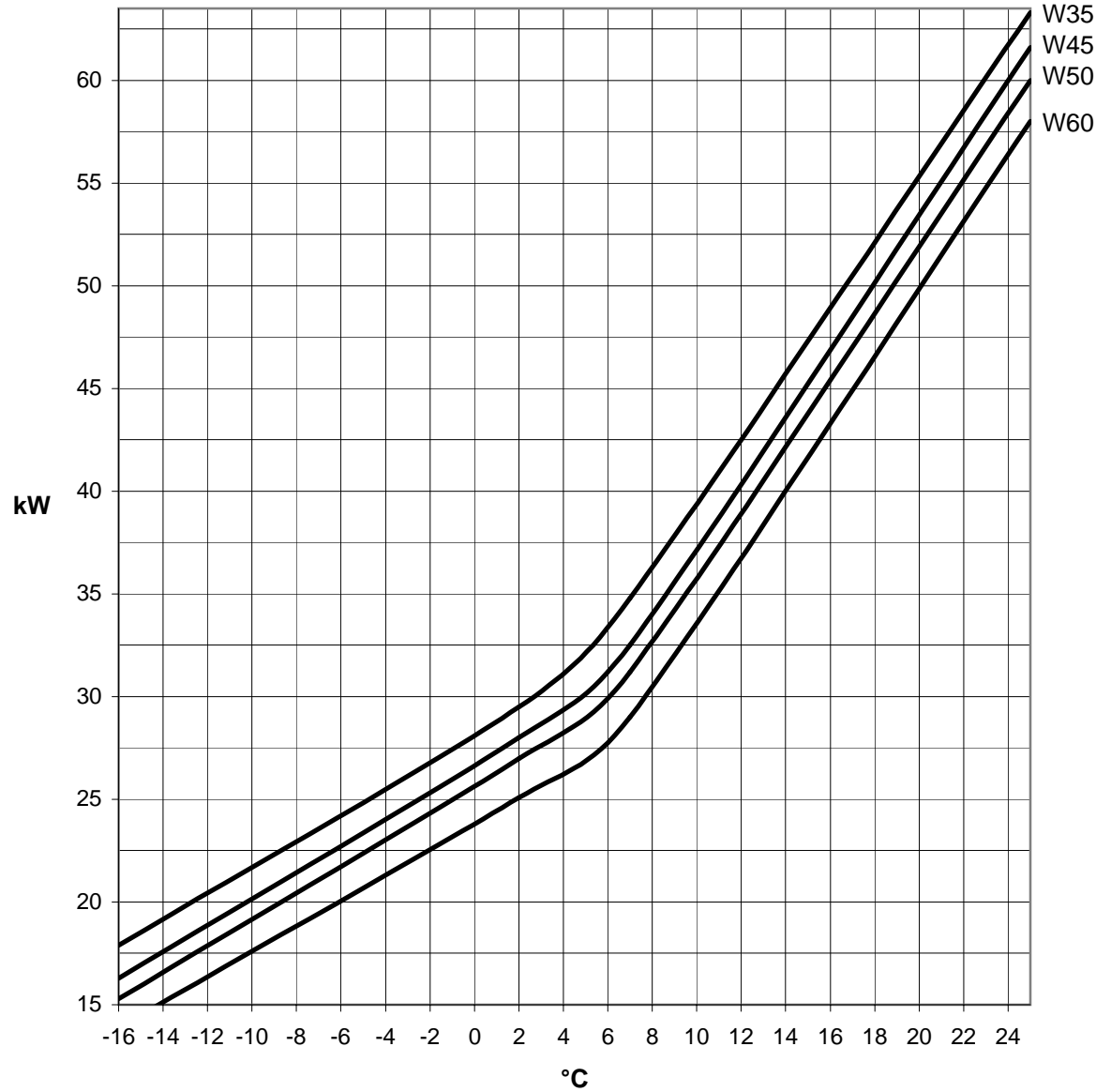
Heizleistung GMLW 35 plus
