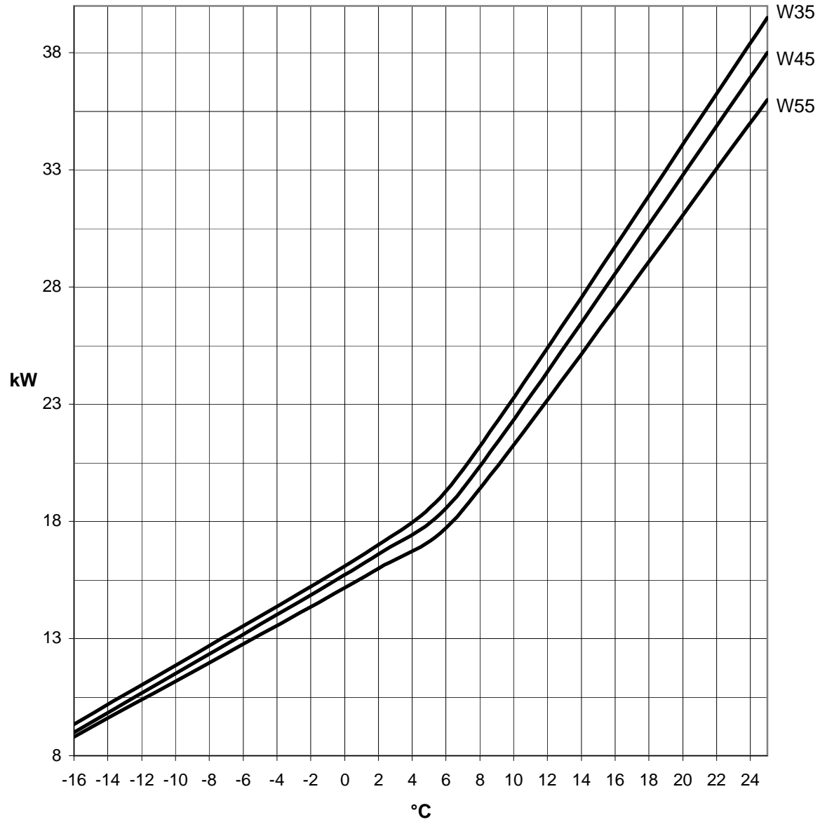
Heizleistung GMLW 19
