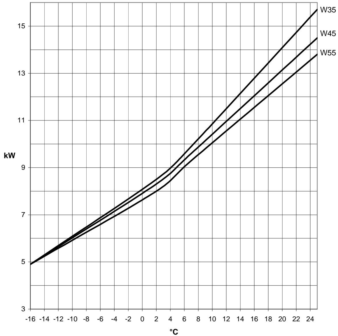
Heizleistung GMLW 9
