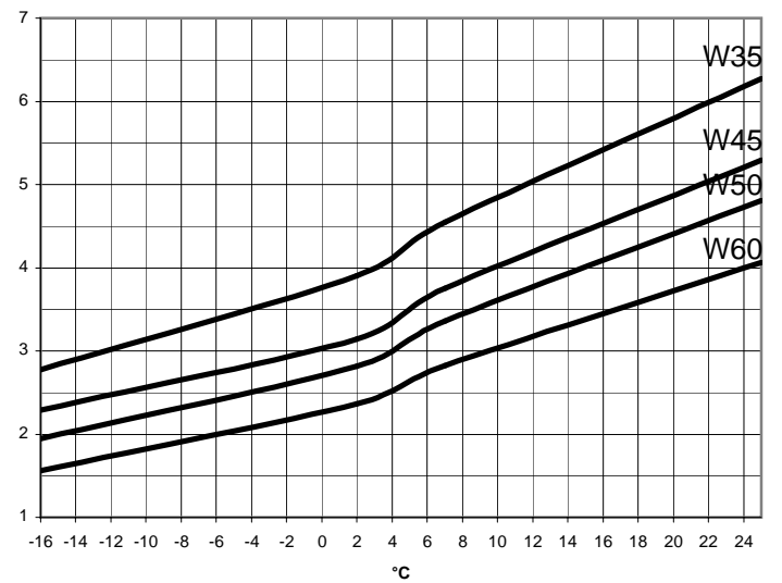
Leistungszahl GMLW 14 plus
