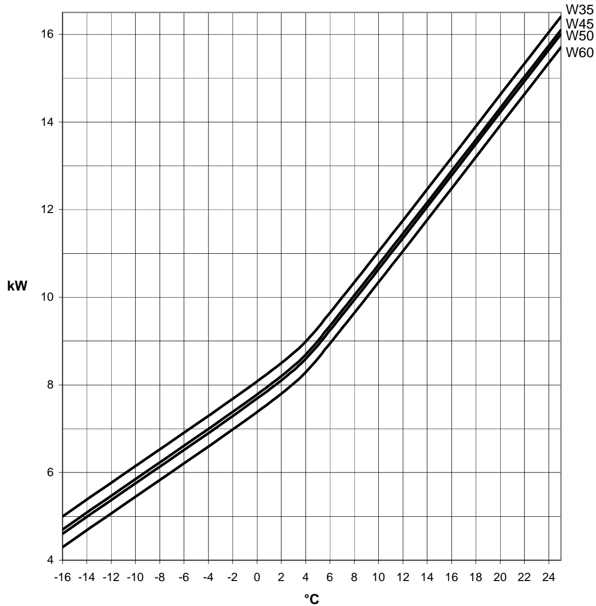
Heizleistung GMLW 9 plus
