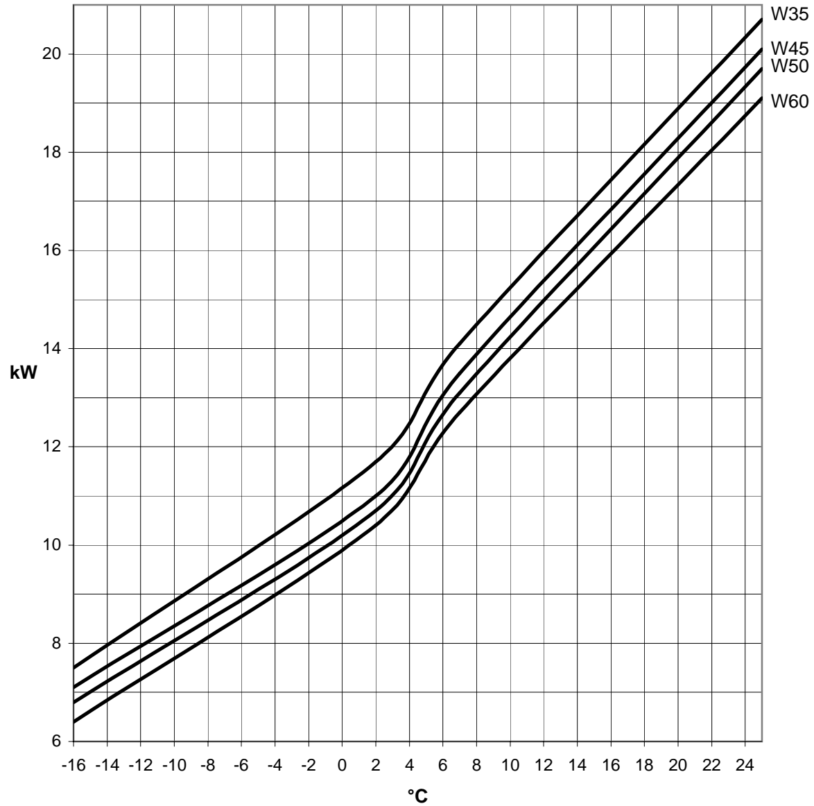
Heizleistung GMLW 14 plus
