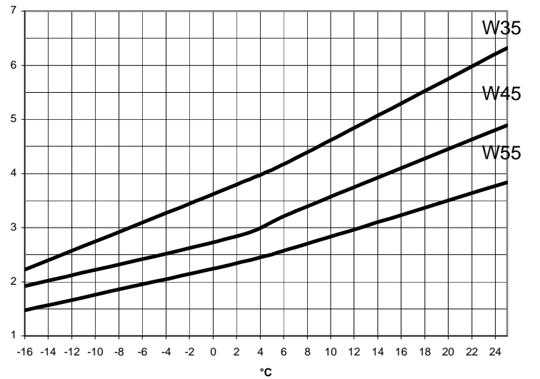
Leistungszahl GMLW 25
