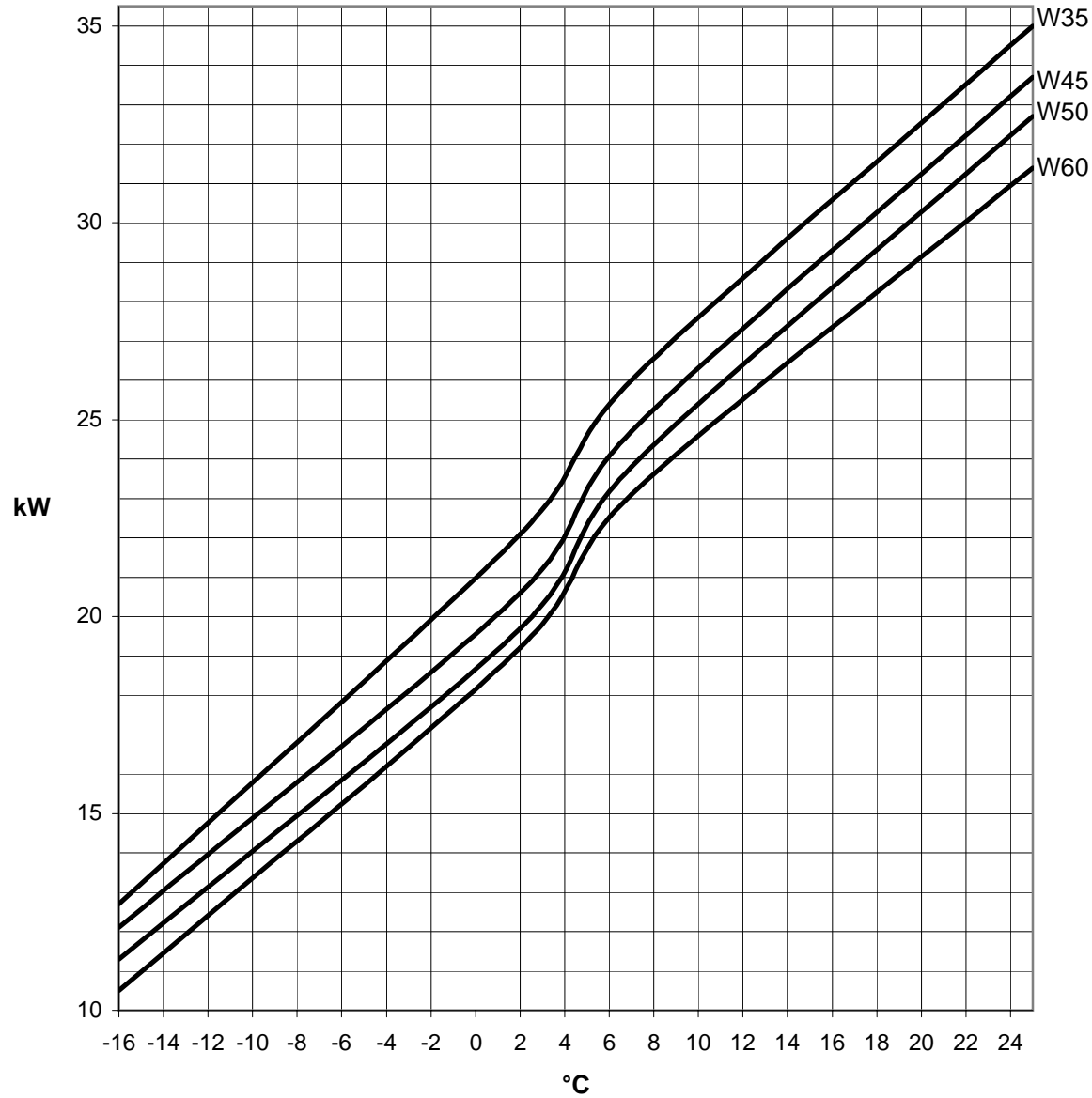
Heizleistung GMLW 25 plus
