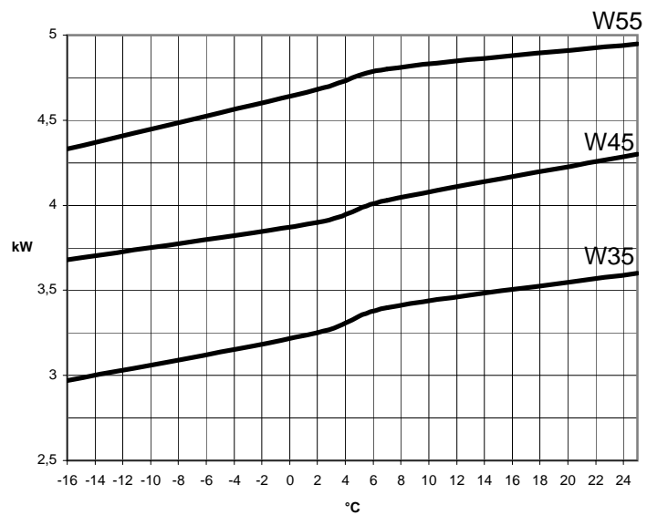
Leistungsaufnahme GMLW 14
