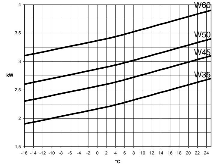
Leistungsaufnahme GMLW 9 plus
