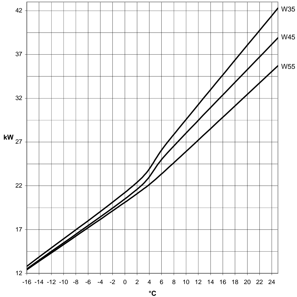
Heizleistung GMLW 25
