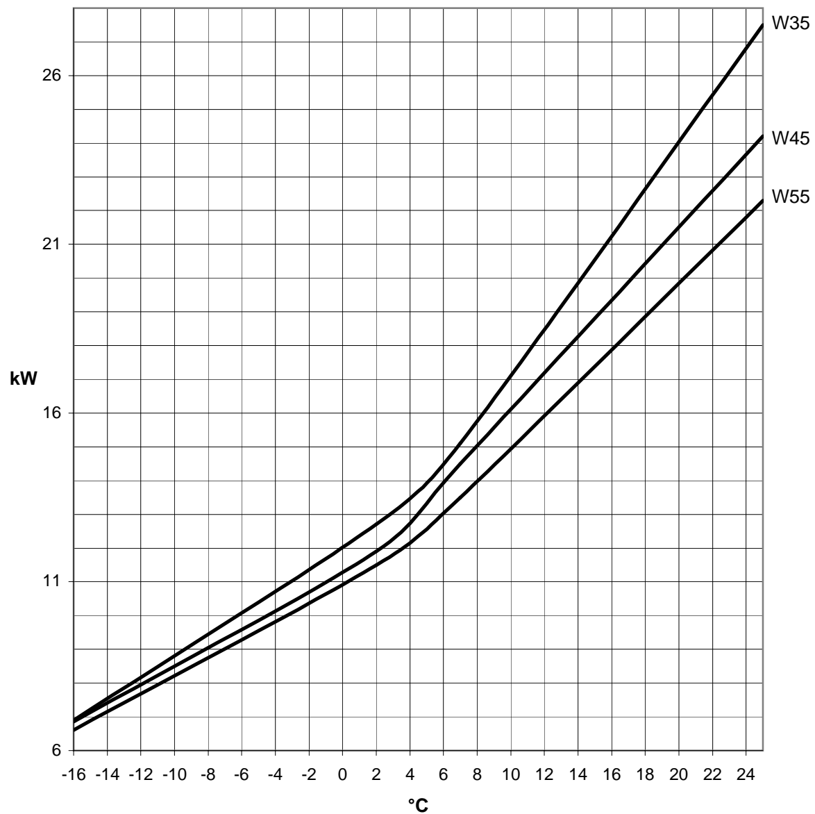
Heizleistung GMLW 14
