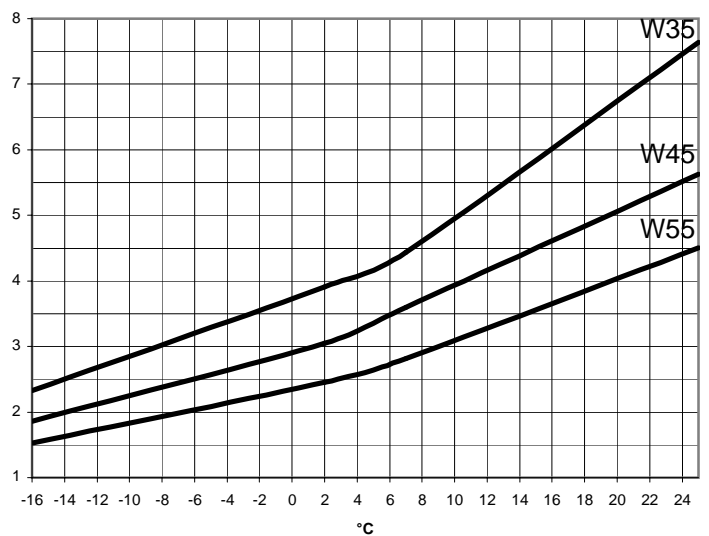
Leistungszahl GMLW 14
